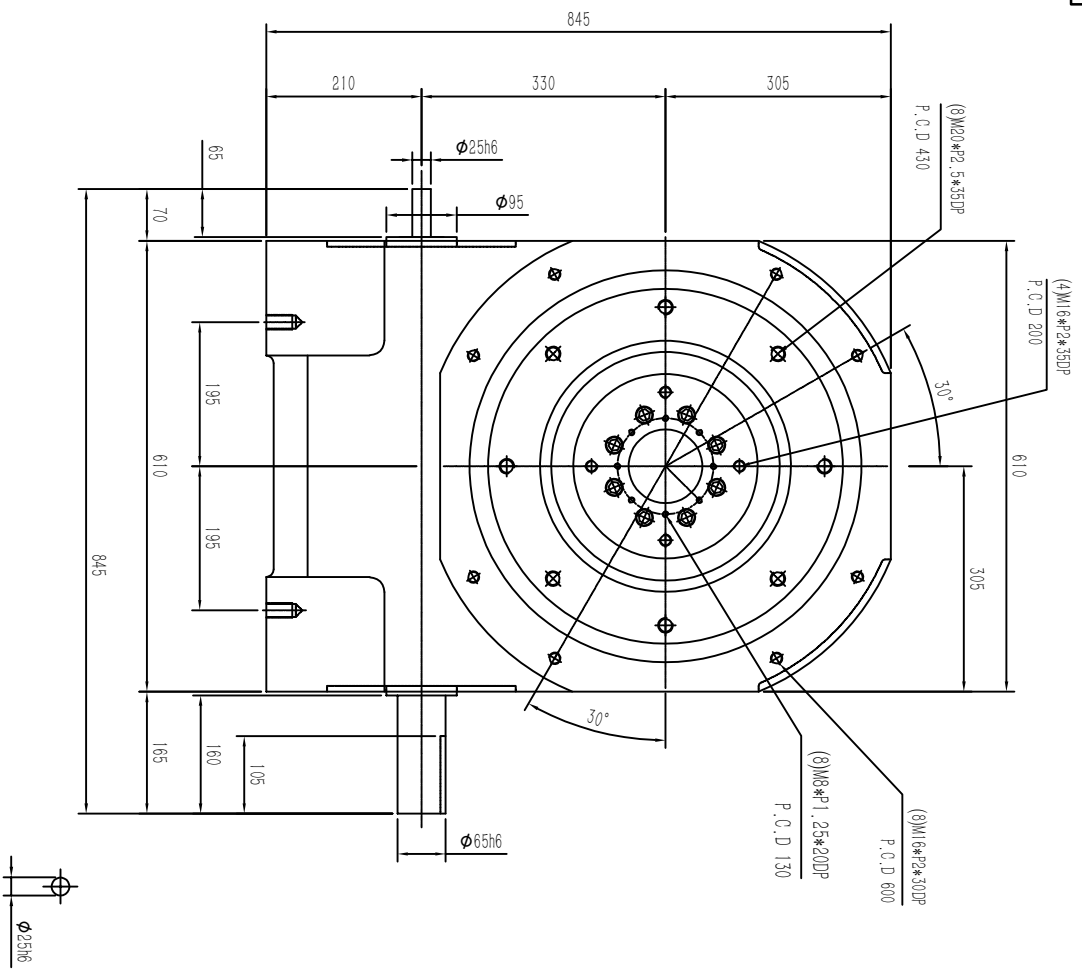
側入力軸
